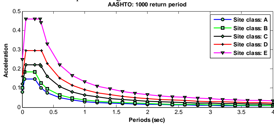
Fig. 2.13 Design spectra: AASHTO 1000 yr. return period
